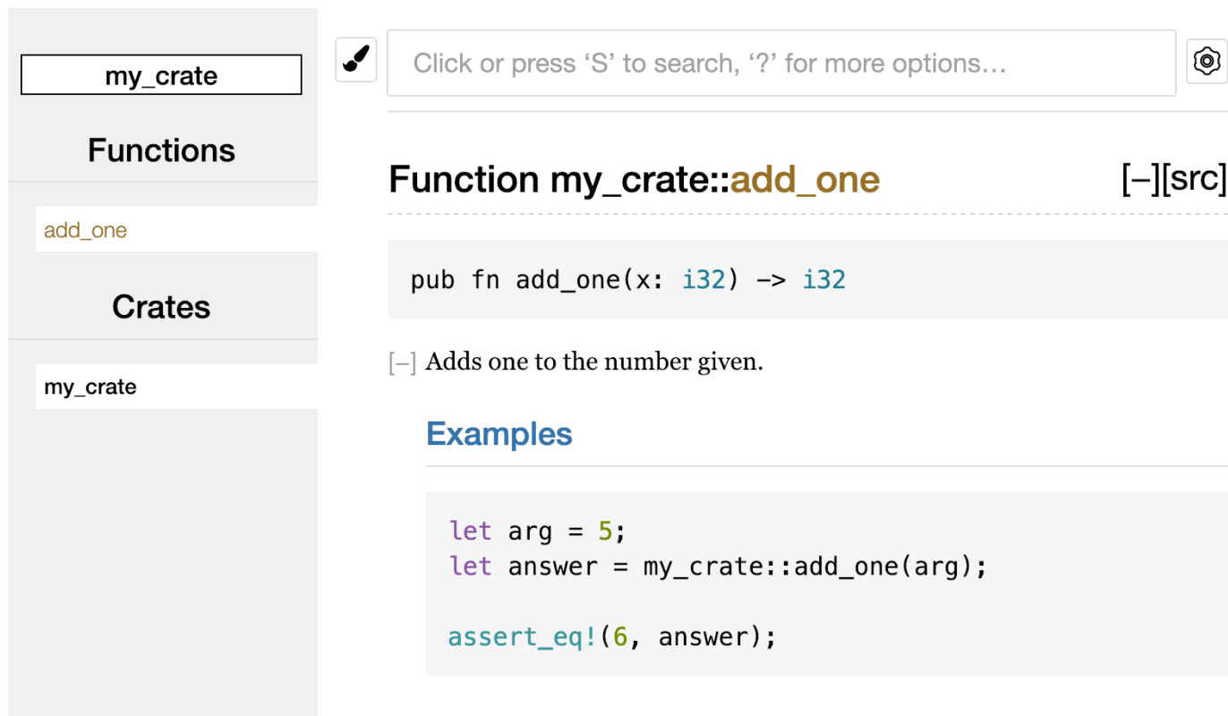
图 14-1: add_one 函数的文档注释 HTML
