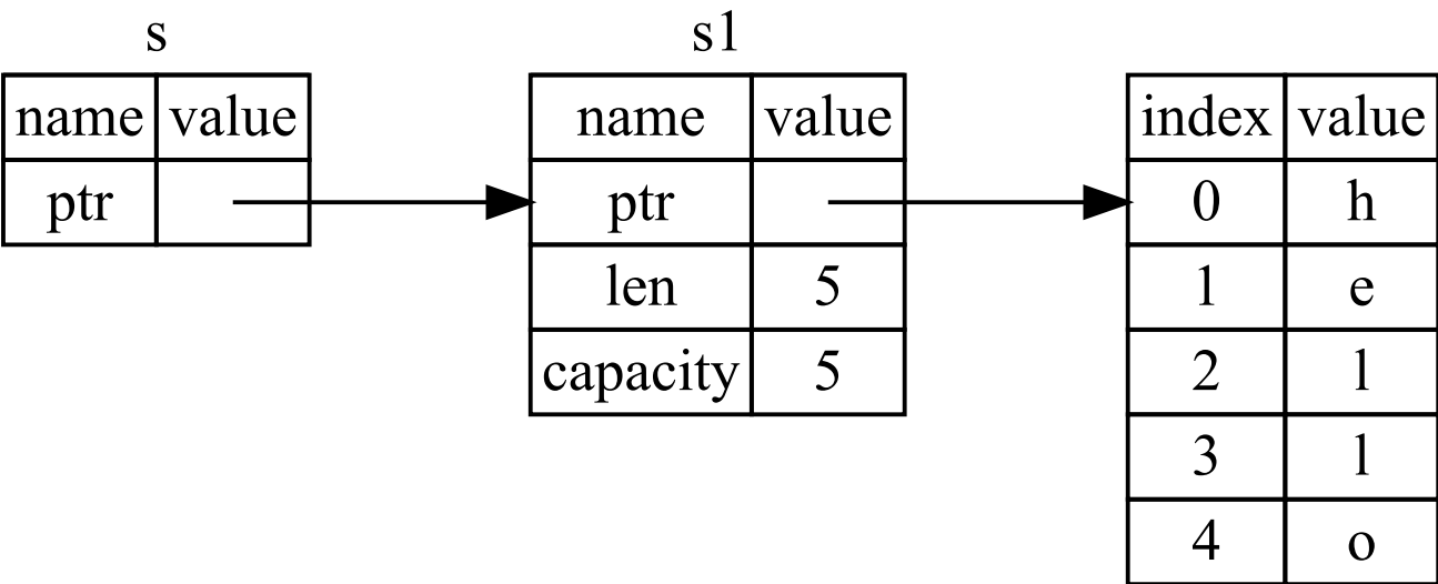
图 4-5: &String s 指向 String s1 示意图
